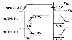
TTL INTERFACE
