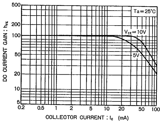
Fig. 5 直流電流増幅率—コレクタ電流特性 (I)
