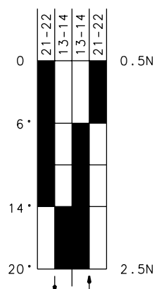
Schaltdiagramm Schaltsymbol
