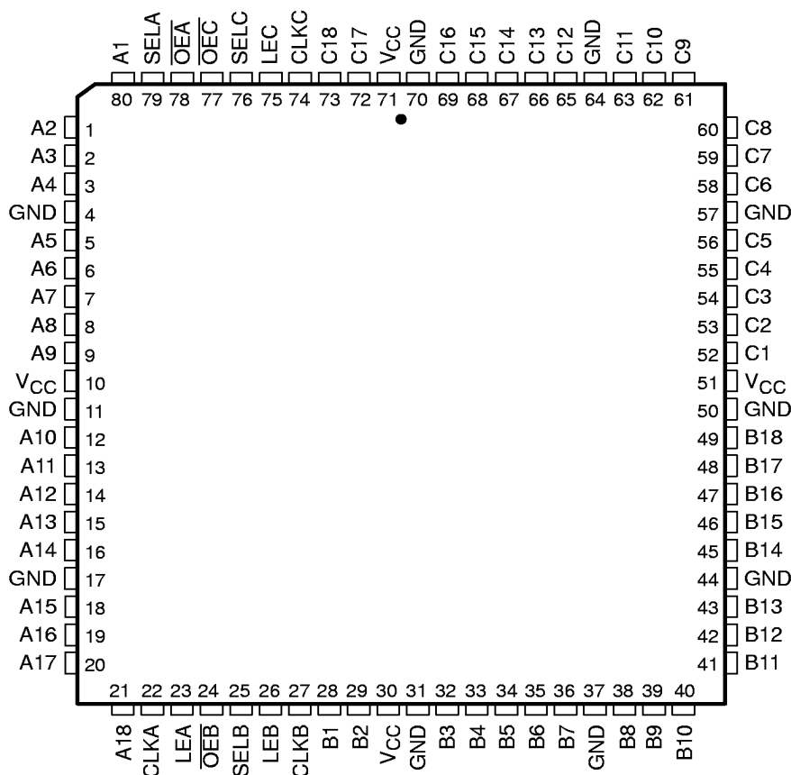
SN74ABTH32318 . . . PN PACKAGE (TOP VIEW)
