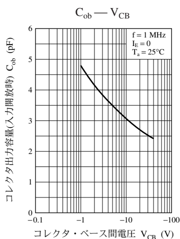
UNR4116 特性図
