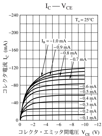
UNR4119 特性図
