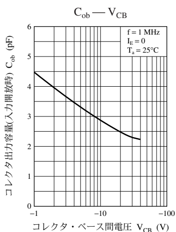
UNR411M 特性図
