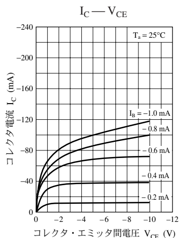
UNR411L 特性図
