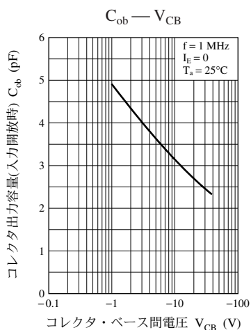
UNR4119 特性図
