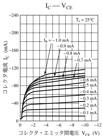
UNR4118 特性図
