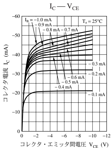
UNR411E 特性図
