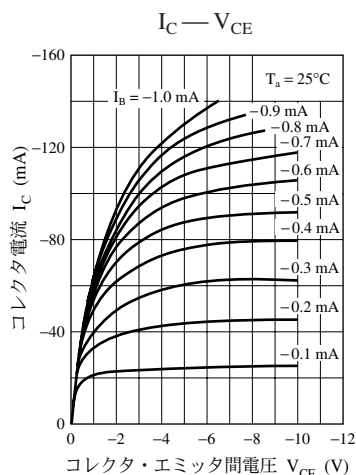
UNR4115 特性図
