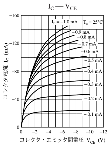
UNR4113 特性図
