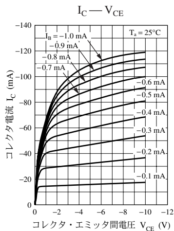
UNR411M 特性図
