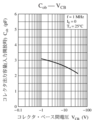
UNR411F 特性図
