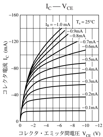
UNR4112 特性図
