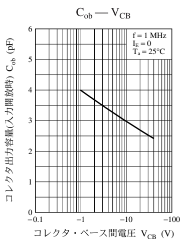
UNR4113 特性図
