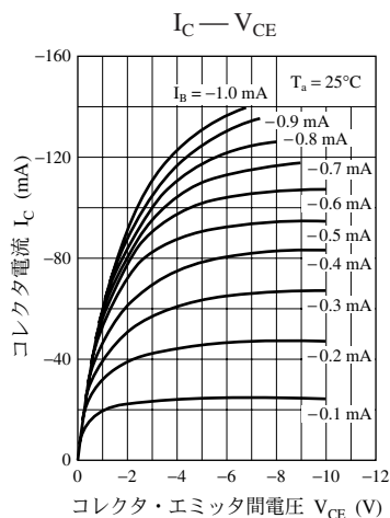
UNR4116 特性図
