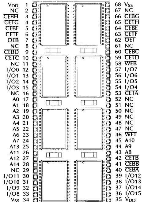
DPS96122
