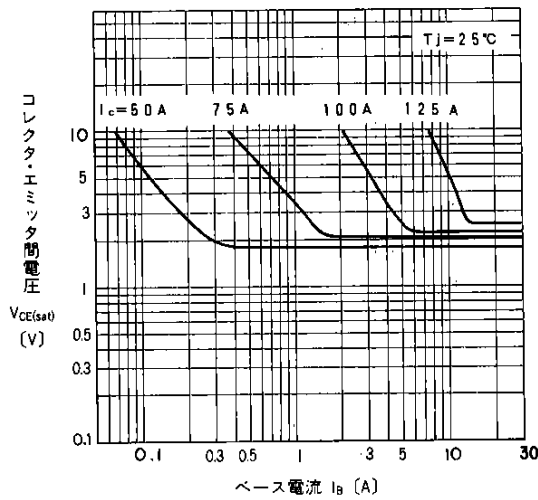
出力特性
