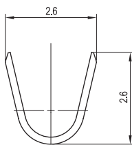
SEC A-A'
