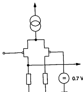
Fig. 3-12: Input Pin 30
