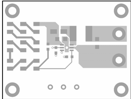
Figure 2—Top Layer
