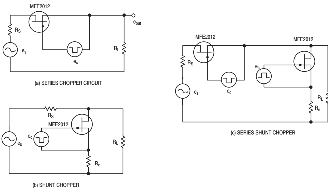
Figure 23. FET Chopper Circuits
