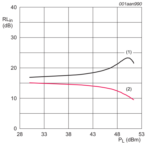
V_{DS} = 28\text{ V}; I_{Dq} = 1300\text{ mA}. (1) f = 2110\text{ MHz} (2) f = 2170\text{ MHz}
