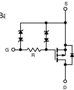
P-Channel MOSFET
