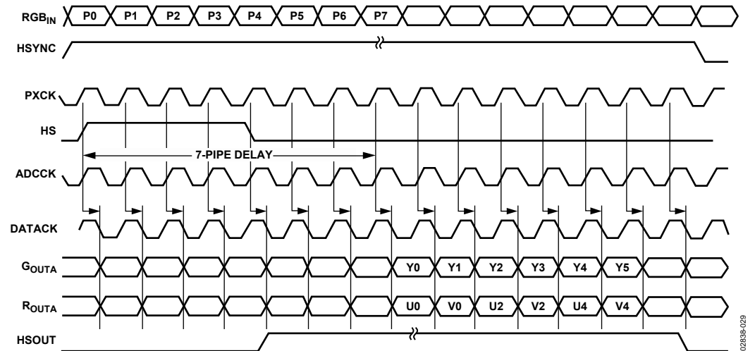
Figure 27. 4:2:2 Output Mode
