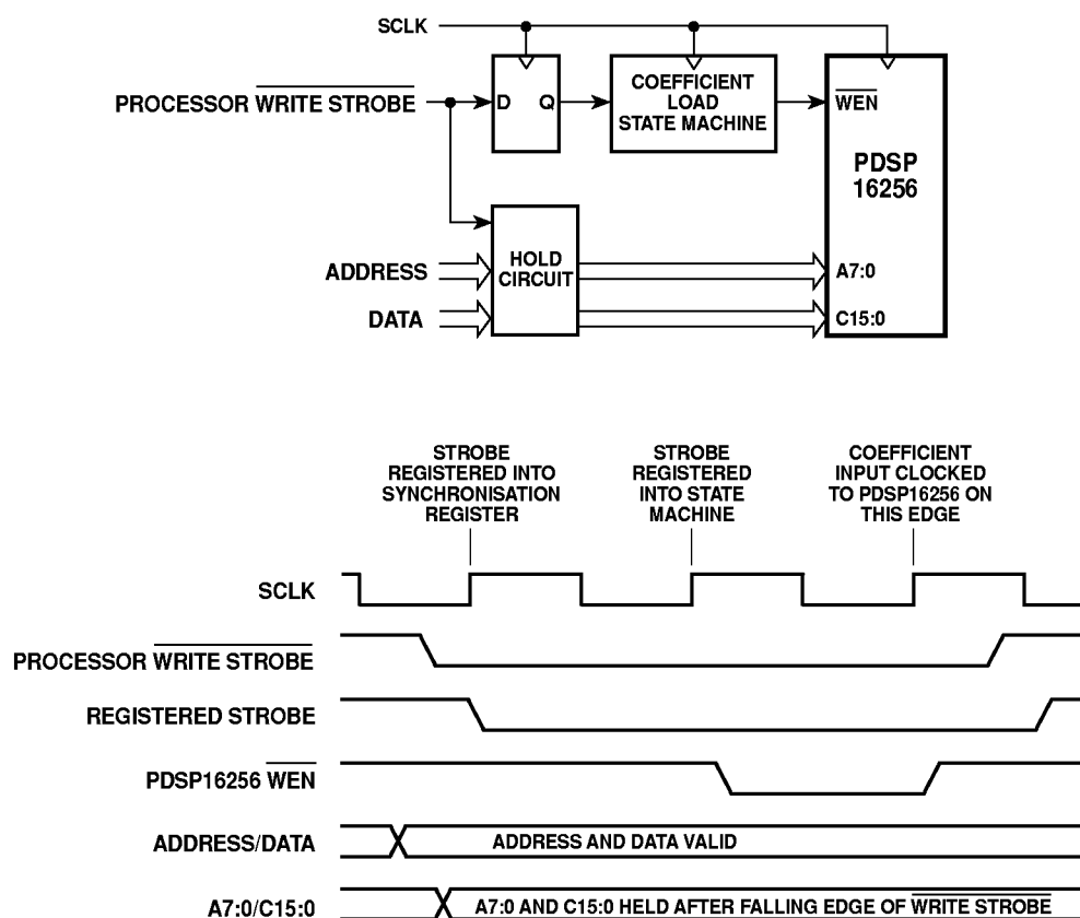
Fig. 18 Remote Master synchronisation
