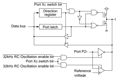
(10) Port P20
