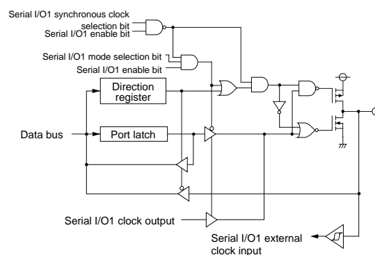
(16) Port P26
