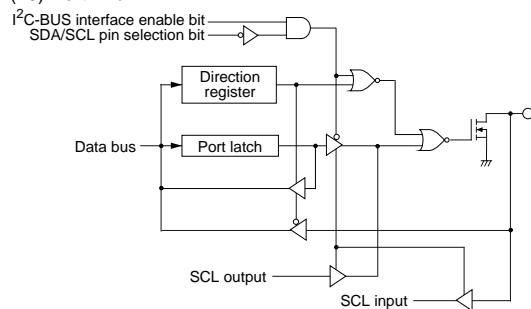
(13) Port P23
