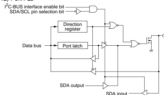
(12) Port P22
