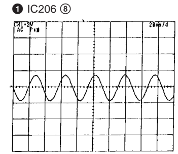
3.28 Vp-p 27 MHz
