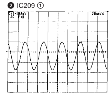
1.4 Vp-p 27 MHz
