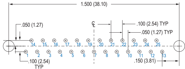
25 SOCKET M83513/25-D
