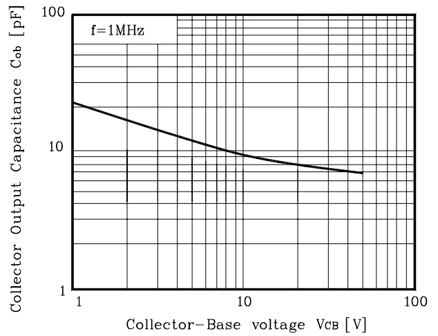
Fig. 4 C_{ob} - V_{CB}
