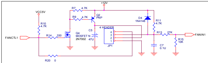
(4 PIN FAN Control) PWM FAN 1 SPEED CONTROL
