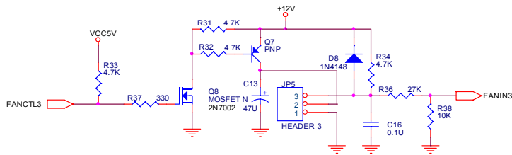
PWM FAN 3 SPEED CONTROL
