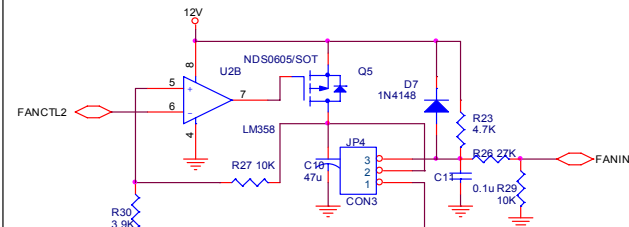
DC FAN Control with OP 2
