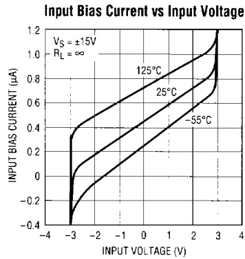
LT1203/05 • TPC13
