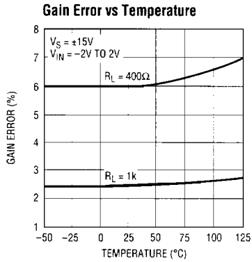
LT1203/05 • TPC12
