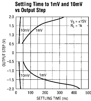
LT1203/05 • TPC15
