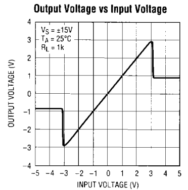
LT1203/05 • TPC14
