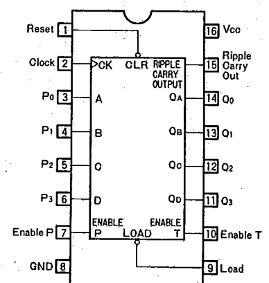
Fig. 38 BU74HC160
