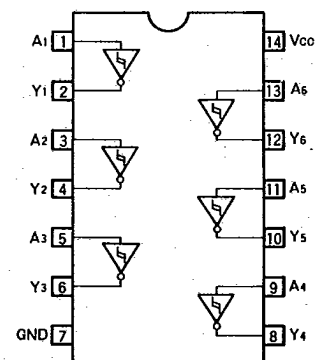
Fig. 22 BU74HC14
