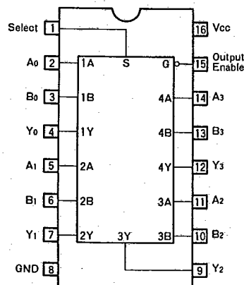
Fig. 34 BU74HC157
