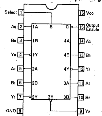
Fig. 35 BU74HC158
