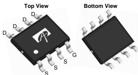
SOIC-8
