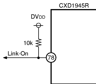
Fig. 3-7. CMC/LINKON Pin when CMC = 1
