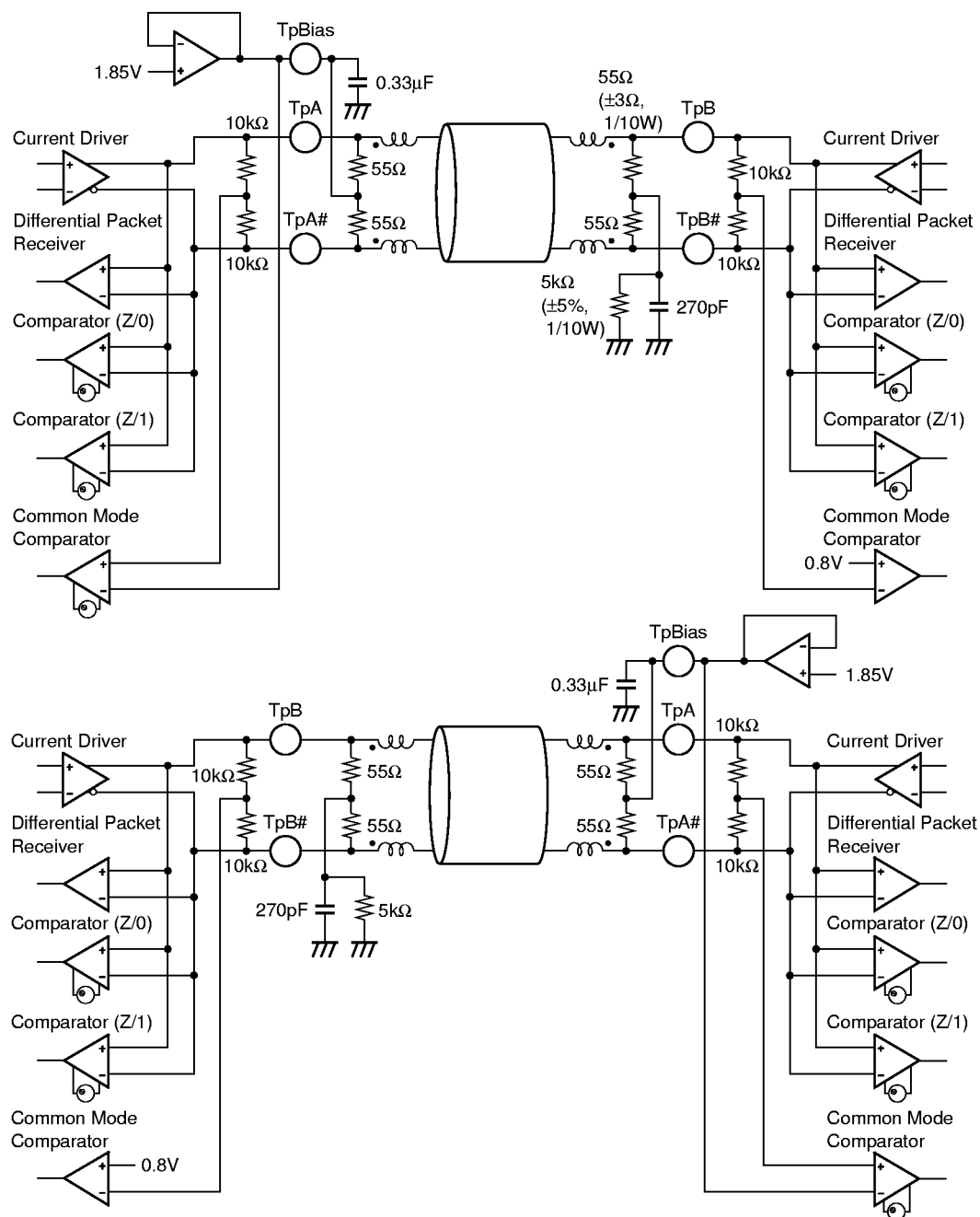
Fig. 3-9. Cable Interface
