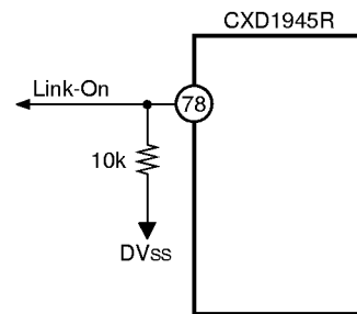
Fig. 3-8. CMC/LINKON Pin when CMC = 0
