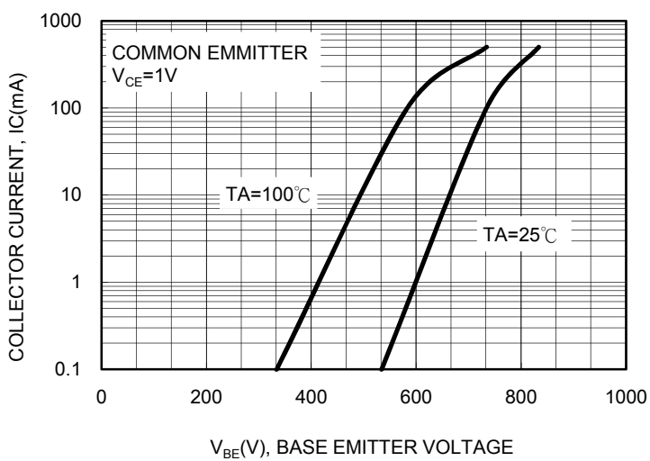
FIG. 5 I_C - V_{BE}
