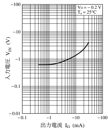
V_{IN} - I_O
