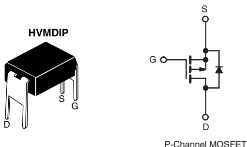
P-Channel MOSFET
