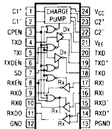
DTE LTC1323
