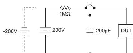
ESD test
