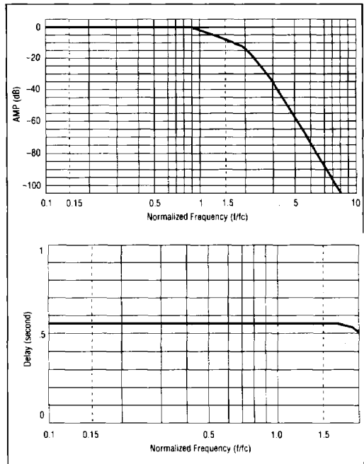
Bessel
