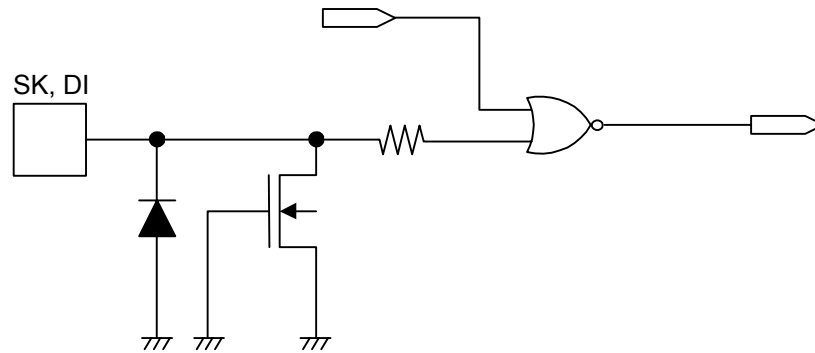
Figure 23 SK, DI Pin
