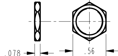
2X HEX NUT 3
