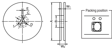
Reel dimensions
