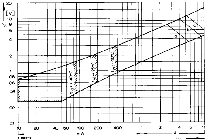
Bild/Fig. 19 Steuercharakteristik mit Zündbereichen/Gate characteristic with triggering areas V_G = f(i_G) , V_D = 6 \text{ V} Parameter: Steuerimpulsdauer/Trigger pulse duration t_g [ms] 10 1 0,5 Höchstzulässige Spitzensteuerverlustleistung/ Max. rated peak gate power dissipation P_{GM} [W] 20 40 60
