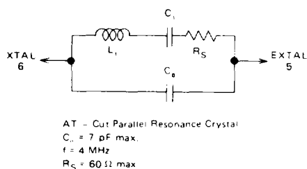
Figure 10 Crystal Parameters
