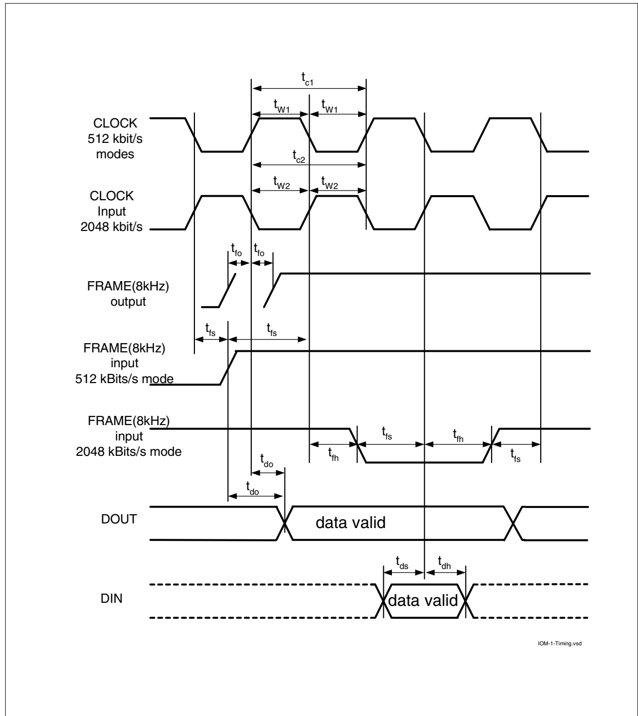
Figure 91 IOM ® -1 Timing
