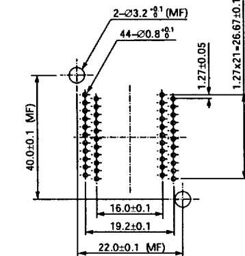
SOP IC51-0442-1315 (44 Pins)
