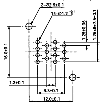
SOP IC51-0142-951 (14 Pins)
