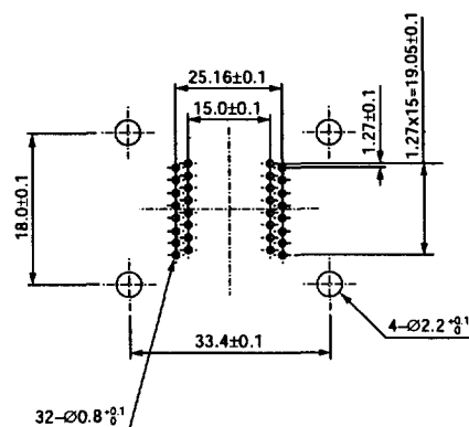
SOP IC51-0322-950 (32 Pins)
