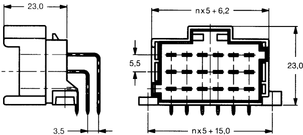
90°-Messerleiste / Tab Header, 90°
