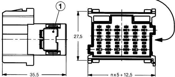
Flachstecker-Gehäuse / Tab Housing
