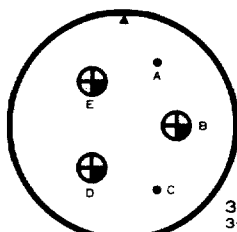
32-1 2-#0, 3-#12 定格-E(A) D(その他)
