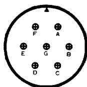
16S-1 7-#16 Serv. A
