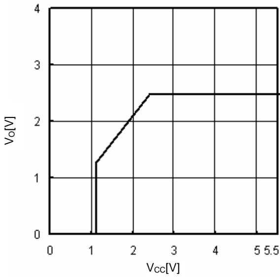
Fig.15 V_{cc}-V_o ( I_o=0mA )
