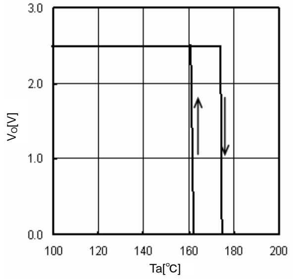
Fig.16 TSD ( I_o=0mA )
