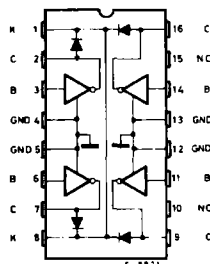
ULN2064B ULN2066B
