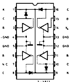
ULN2068B ULN2070B
