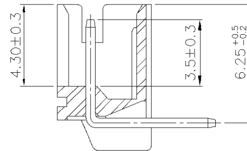
SEC. A-A
