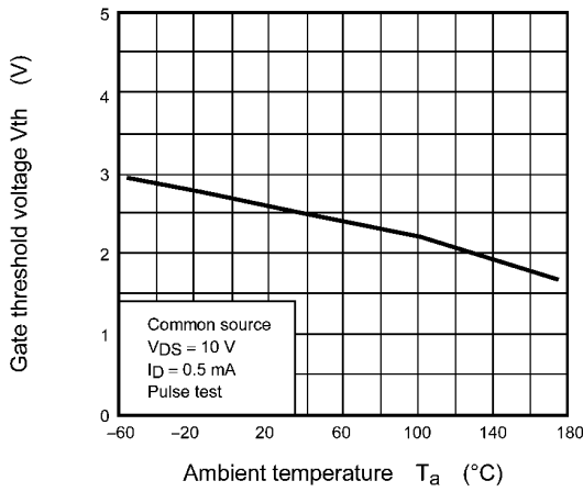
Fig. 8.9 V_{th} - T_a (Note 7)
