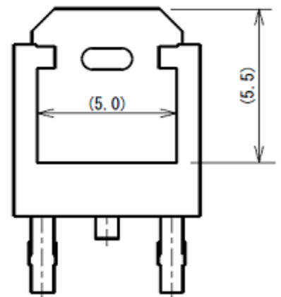
裏面 フィン詳細図
