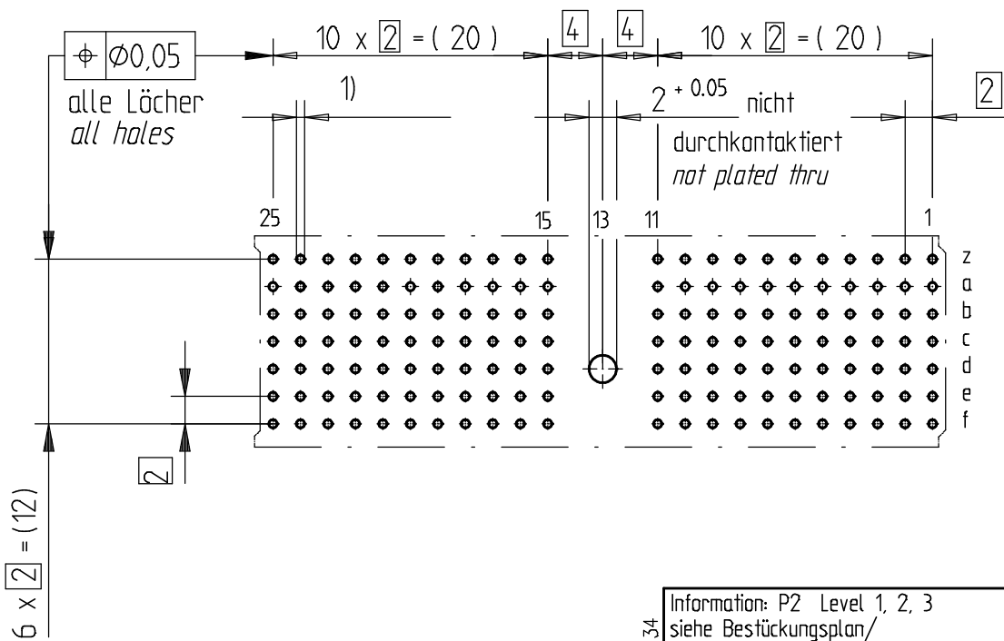
Lochbild für Leiterplatte (Bestückungsseite)
