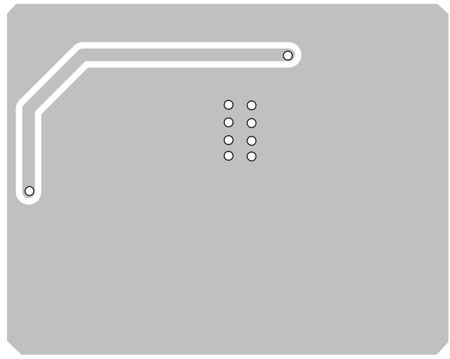
Bottom Layer
