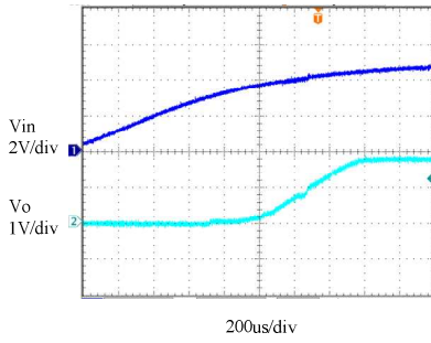
Soft Start(Vo)
