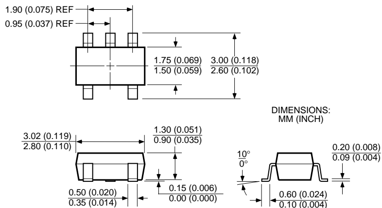
SOT-23-5 (M5)
