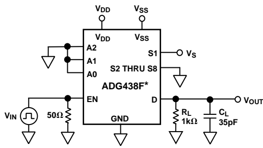
Test Circuit 9. Enable Delay, t_{ON} (EN), t_{OFF} (EN)
