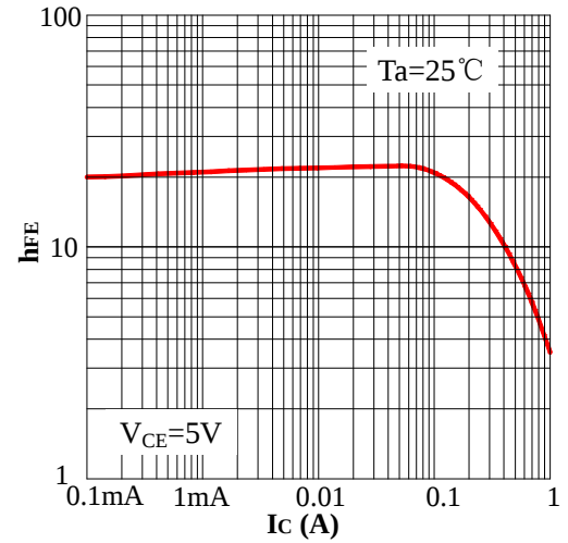
Fig2 h_{FE}-I_C
